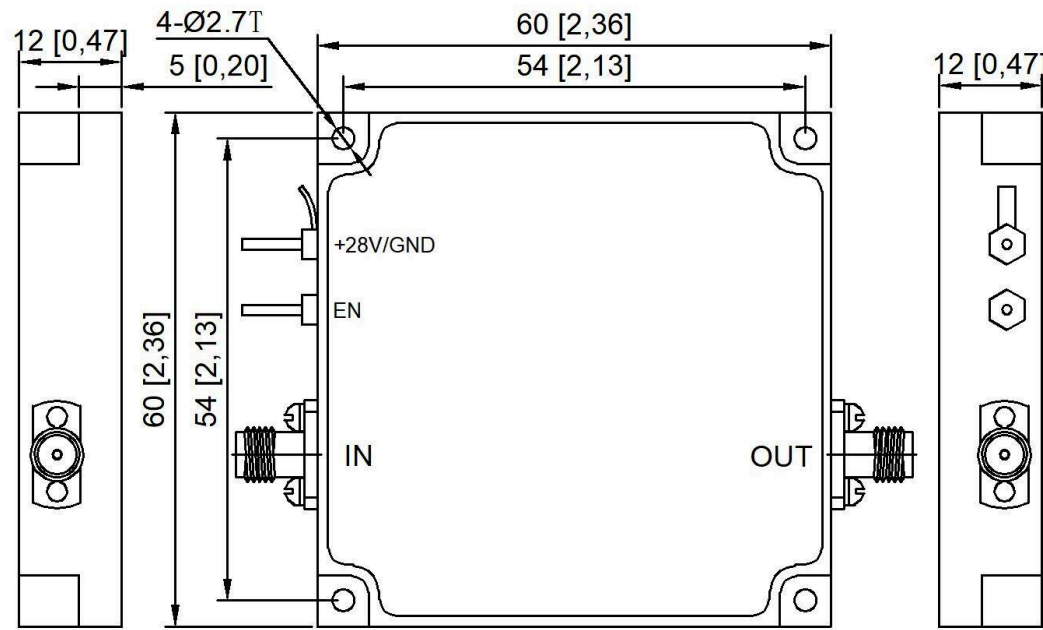
机械外形尺寸图
