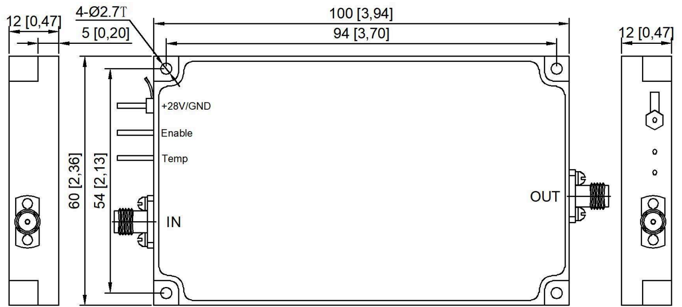
机械外形尺寸图
