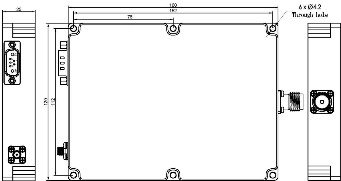
Все размеры указаны в мм [дюймах].
